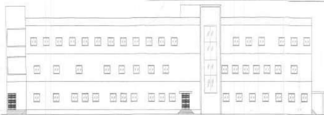
ELEVATION SCALE: 1/50
